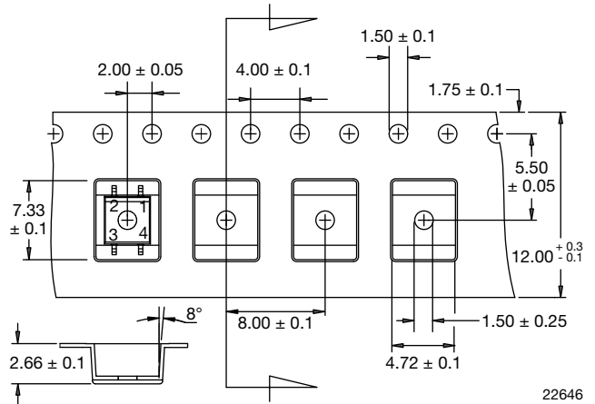
Fig. 11 - Tape Dimensions
