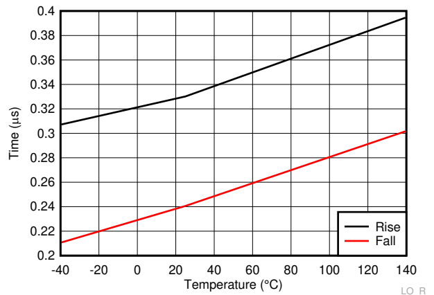
Figure 6-24. HO Rise Time
