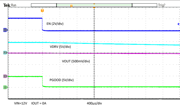
Figure 8-11. EN Shutdown
