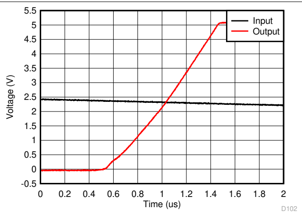
Figure 10-5. Rising Edge
