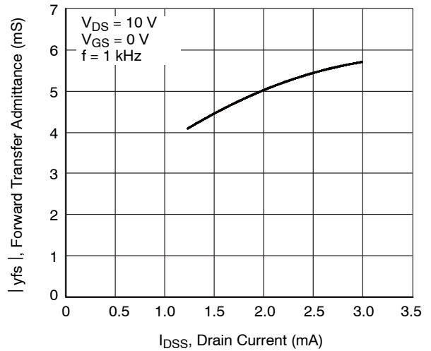
Figure 6. |y_{fs}| - I_{DSS}
