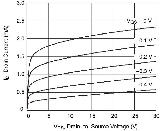
Figure 2. I_D - V_{DS}
