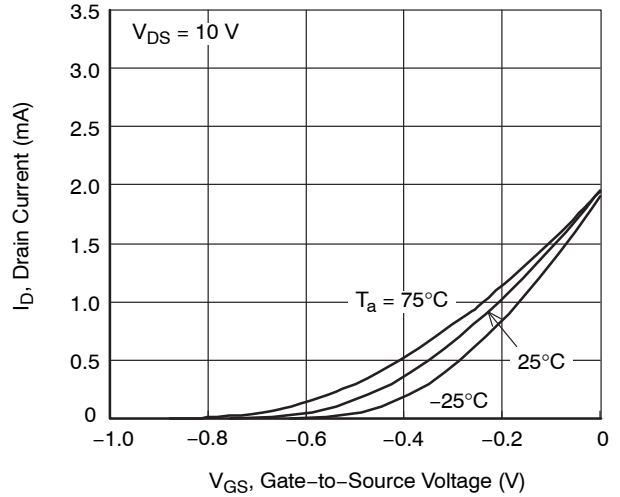
Figure 4. I_D - V_{GS}
