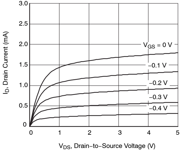
Figure 1. I_D - V_{DS}
