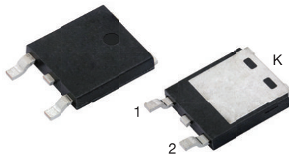
SlimDPAK (TO-252AE)
