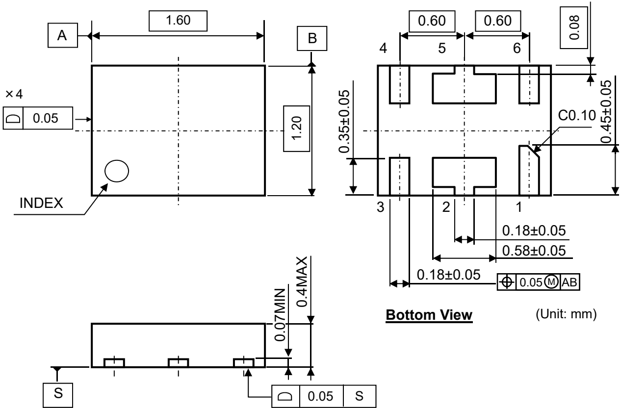
DFN(PL)1216-6G Package Dimensions
