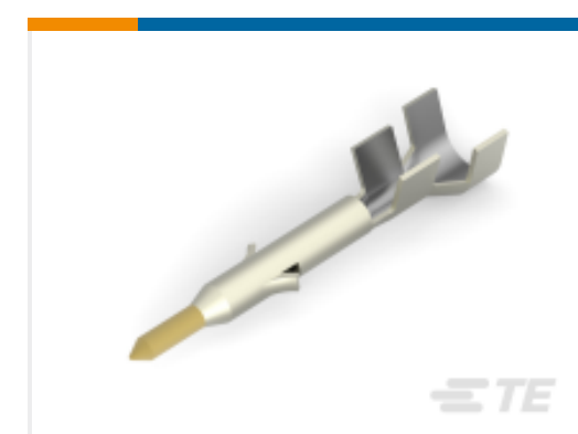
TE Part # 1-794406-0 MINI UMNL SOK 20-16 AWG AU LF
