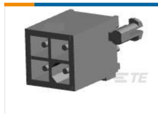
TE Part #1-770174-1 04P MINI UMNL ASSY VO SNAU LF
