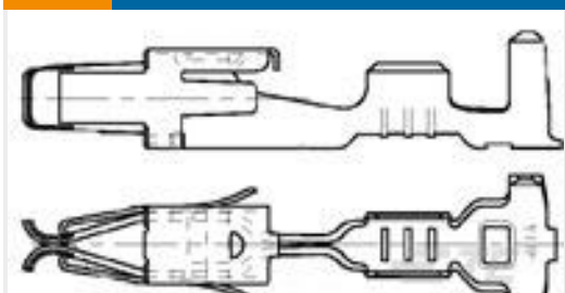
TE Part #5-962885-1 MQS0,63 Sn rec LL EDS 0,2-0,35
