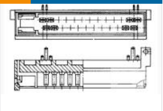
TE Part #826141-1 25 POS TAB HEADER
