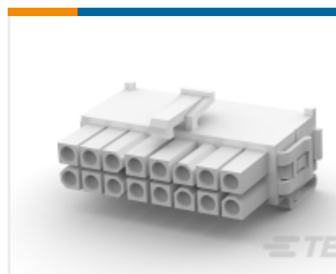
TE Part # 794206-1 16P MINI UMNL2 PLUG HSG UL94V0
