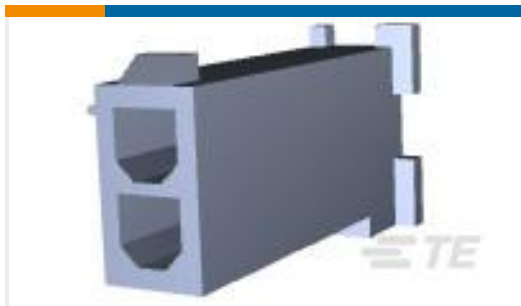
TE Part #172233-1 2 POS MINI UMNL CAP HOUSING
