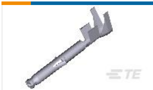
TE Part #770988-3 MINI UMNL SOK 22-18AWG AU LP
