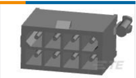
TE Part #794073-2 08P MINI UMNL HDR W/O DH AU
