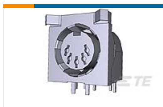
TE Part #5750477-1 5 CIRC DIN RCPT W/GRND FINGERS
