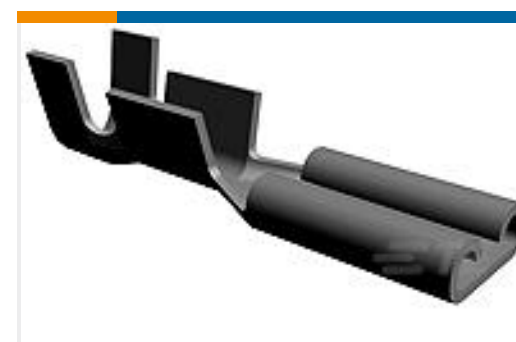
TE Part #63391-1 093 FASTON TAB REC 22-18 AWG TPBR
