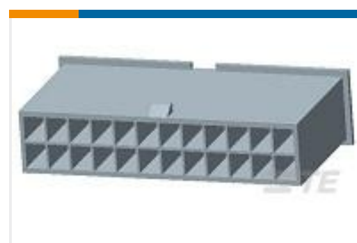
TE Part #1-1969612-0 10P FH PLUG VAL-U-LOK V0
