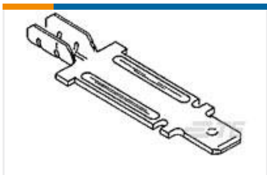
TE Part #63301-1 250 FASTON TAB 22-15 AWG NPST
