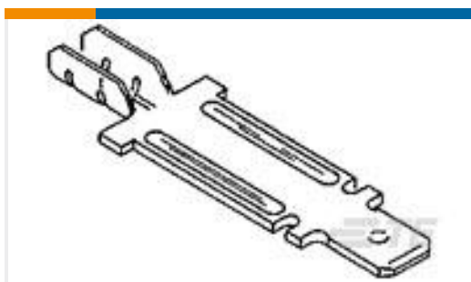
TE Part #63301-1 250 FASTON TAB 22-15 AWG NPST
