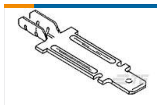
TE Part #63301-1 250 FASTON TAB 22-15 AWG NPST
