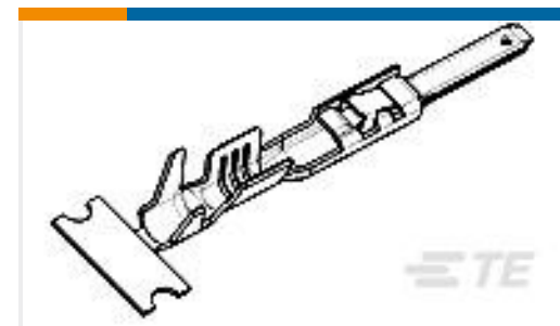
TE Part #1-1452350-1 MQS1,5 Sn tab LL unseal. 0,35-0,5
