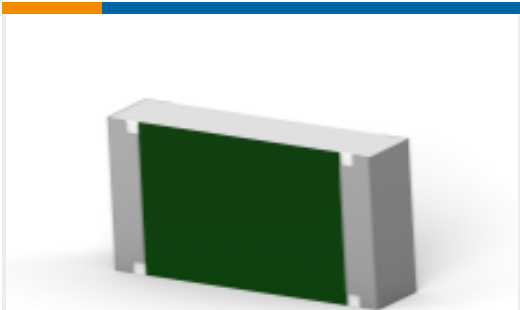
TE Part #2176397-4 3502 1R3 1%
