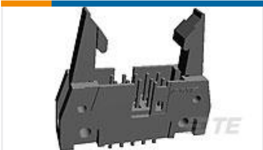
TE Part #2-5499206-1 A/L UNIV HDR 10P VERT LG LAT B
