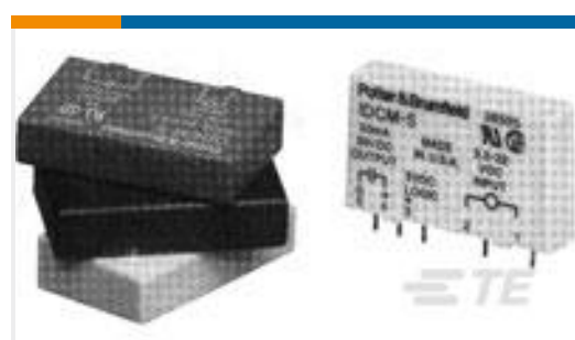
TE Part #5-1393028-1 ODCM-5 = SLIM PCB MOUNT,3A,60V DC-DC I/p
