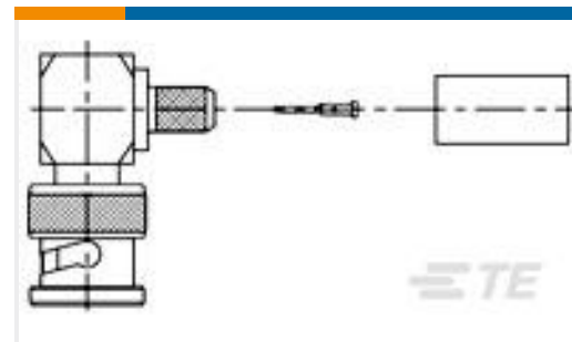
TE Part #1-1337544-0 BNC R/A Plg Hex 50Ohm Nickel Pltd RG58C/
