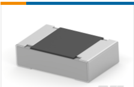
TE Part #3-2176342-7 CRGCQ 0805 1M0 5%
