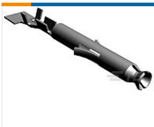
TE Part #770834-1 MINI UMNL SOCKET SN
