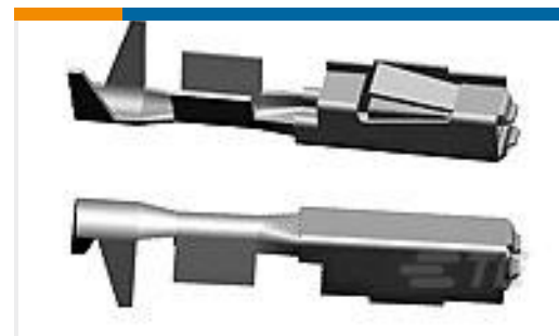
TE Part #144969-1 MQS0,63 Sn rec LL unseal. 0,2-0,6
