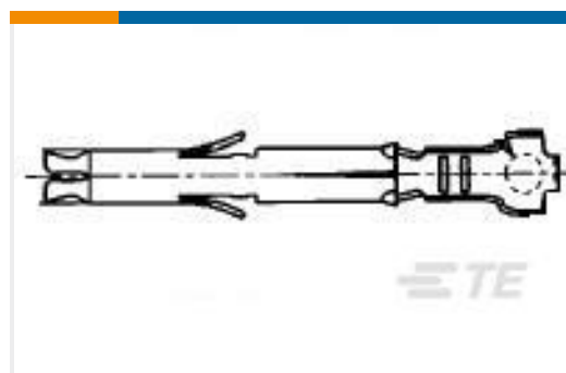
TE Part #170365-1 MINI UNIVERSAL M-N-L SOCKET LP
