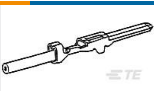
TE Part #175030-1 070 TAB CONTACT L.P 20-16
