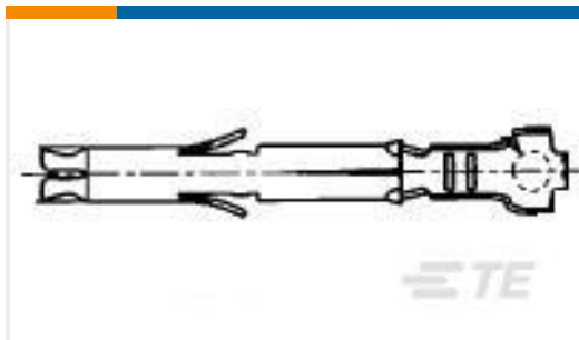
TE Part #170365-3 MINI UNIVERSAL M-N-L SOCKET LP
