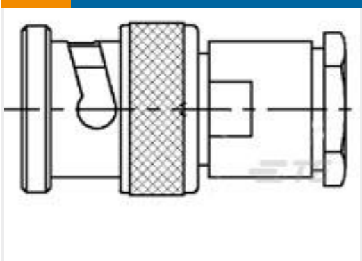
TE Part #1-1337420-0 BNC Str Plg MC 50Ohm Nickel Pltd RG58C/U
