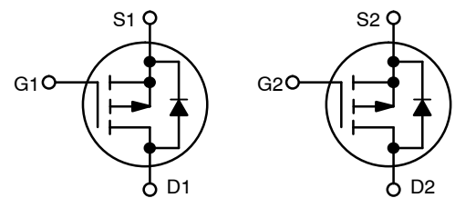
P-CHANNEL MOSFET
