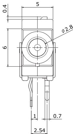
ACTUATOR CAP
