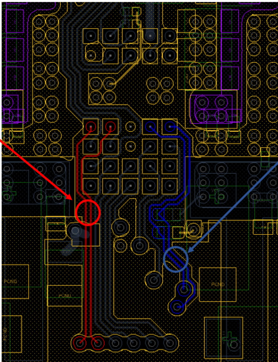
Figure 33 : VSense Traces
