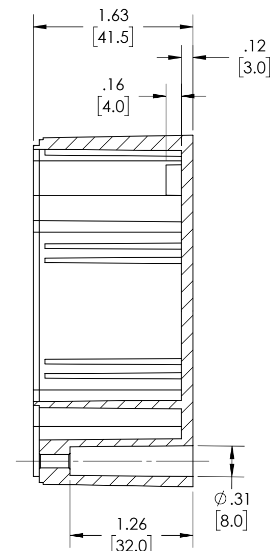
SECTION A-A
