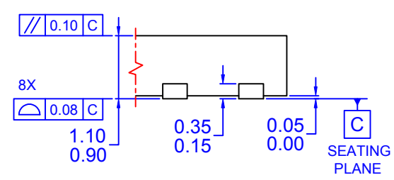
DETAIL 'A' (SCALE: 2X)
