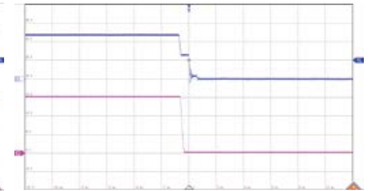
Ch1: Input voltage (10 V/div.) Time scale: (2 ms/div.) Ch2: Output voltage (5 V/div.)
