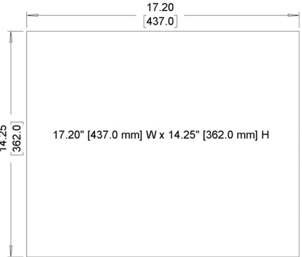
Cutout Dimensions
