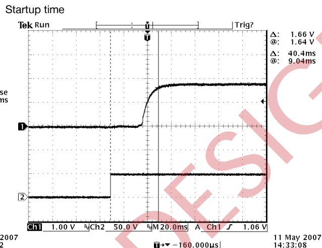
CH1: Vout
