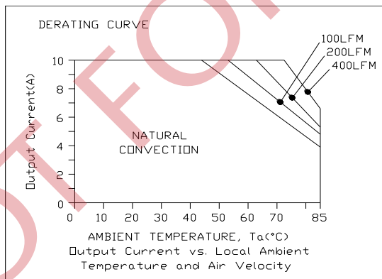
xRSB-40U03x, Vin=18V
