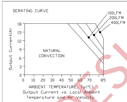
xRSB-40UV2x, Vin=24V
