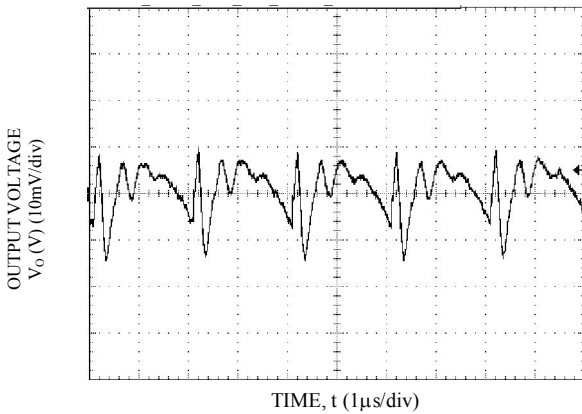
Vo=0.6V, lo = lo,max, Vin=12V
