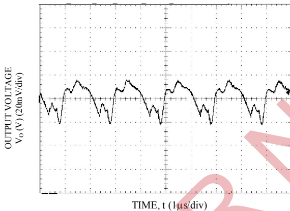
Vo=1.8V, lo = lo,max, Vin=12V
