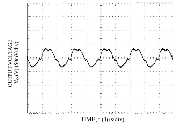
Vo=5.0V, lo = lo,max, Vin=12V
