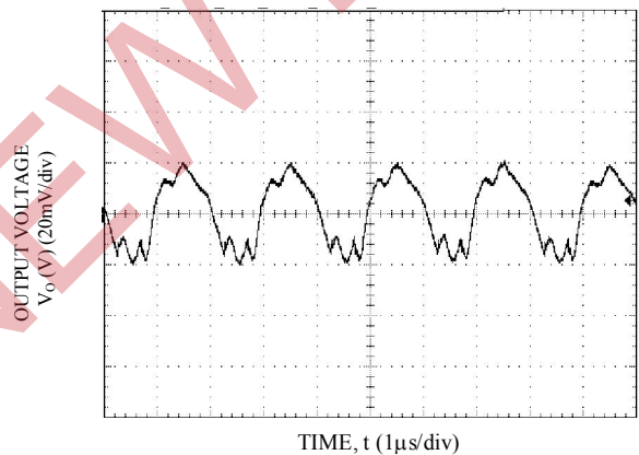
Vo=2.5V, lo = lo,max, Vin=12V
