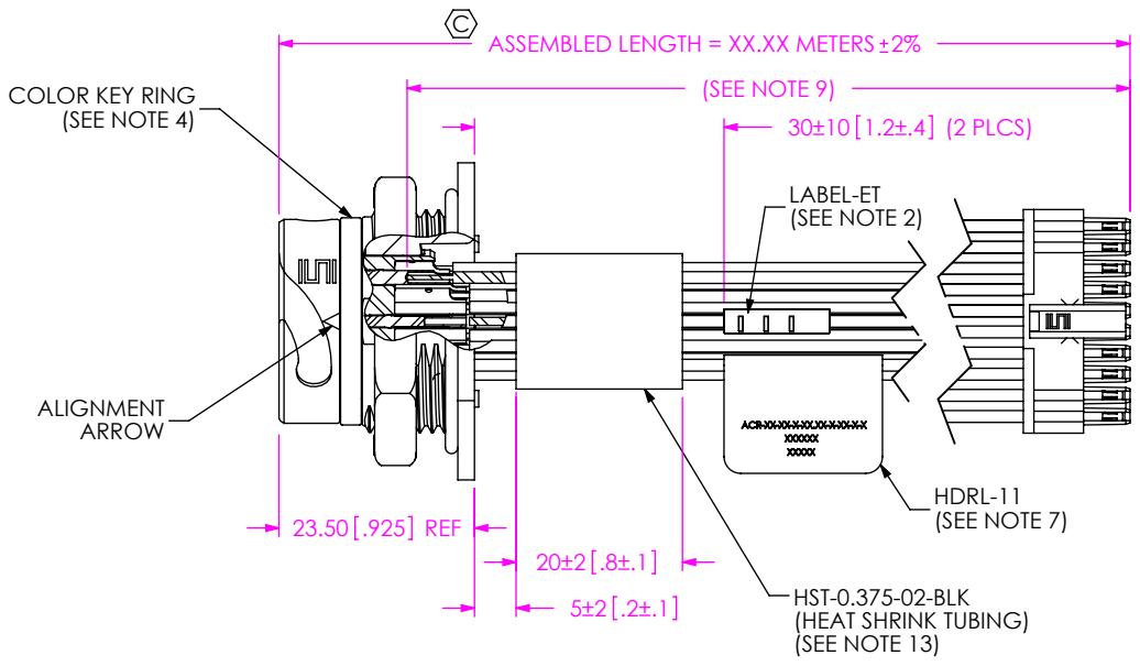
FIG 1 ACR-22-02-X-XX.XX-S-S1-P-1 SHOWN
