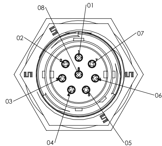
-03: 8 POS ( \varnothing 1.5 SOCKETS)
