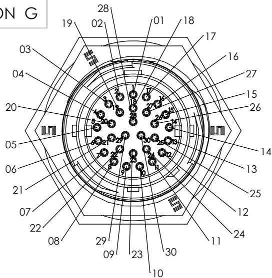
-01: 30 POS ( \varnothing 1.0 SOCKETS)
