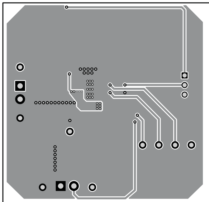
Figure 18. Bottom Layer
