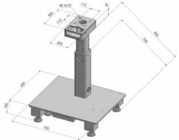
Robot Stand
