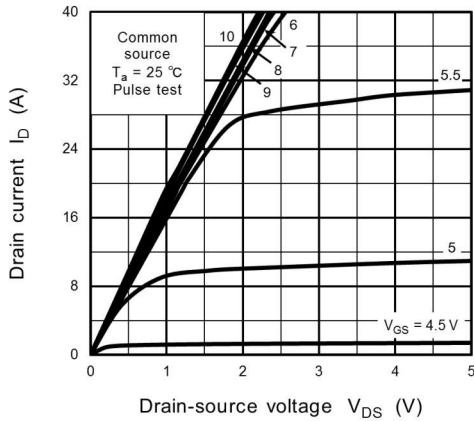
Fig. 8.1 I_D - V_{DS}
