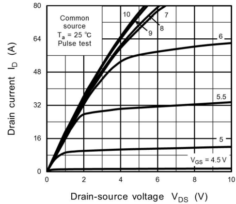
Fig. 8.2 I_D - V_{DS}
