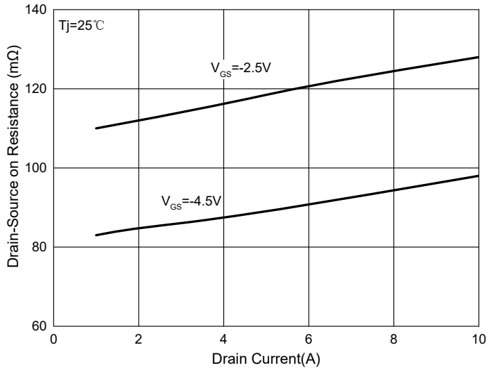
Fig. 7 - R_{DS(ON)} - I_D
