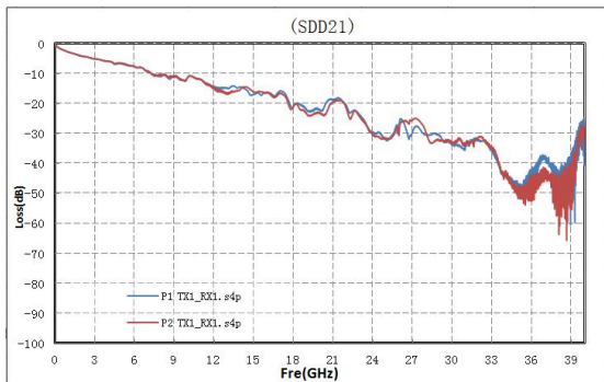
SFP28 26AWG 3M
