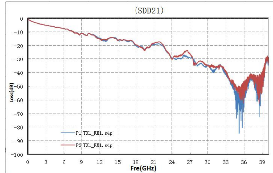
SFP28 30AWG 2M
