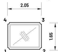
top view crystal pads - 1 & 3 metal lid - 2 & 4
