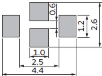
NFM31PC/31KC
