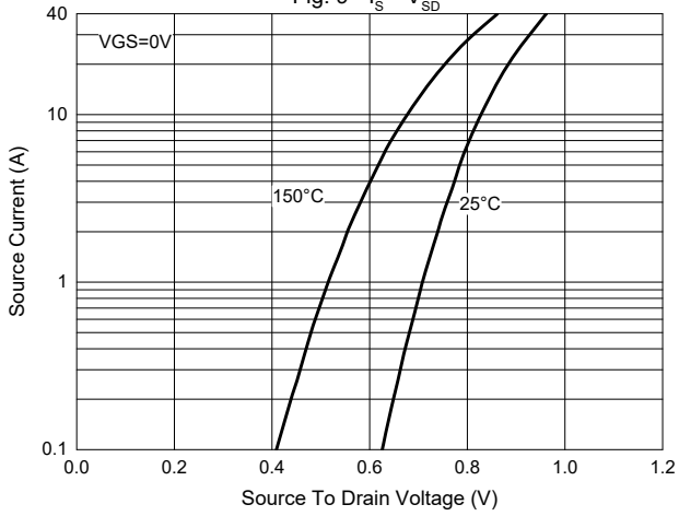
Fig. 9 - I_s - V_{SD}
